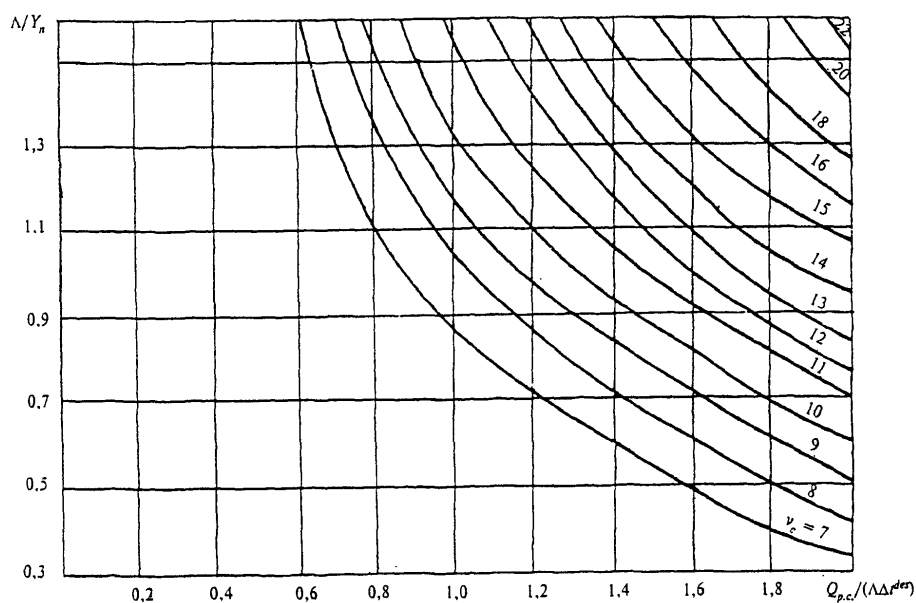
Рисунок 4. График для подбора теплоаккумулирующих приборов (продолжительность зарядки 6 + 2 ч дневной подзарядки)
