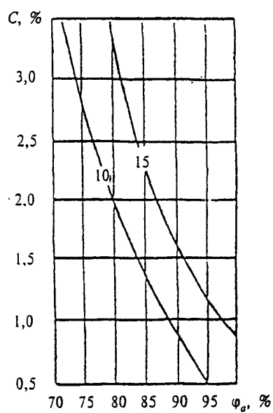
Рисунок Щ.4. Изолинии сорбционного влагосодержания керамзитобетона \rho_0 = 1200 \text{ кг/м}^3 , содержащего NaCl - 60%, KCl - 30%, MgCl_2 - 10%, при изменении относительной влажности воздуха \varphi_a , %, и массового солесодержания C , %, в стенах флото-фабрик.
