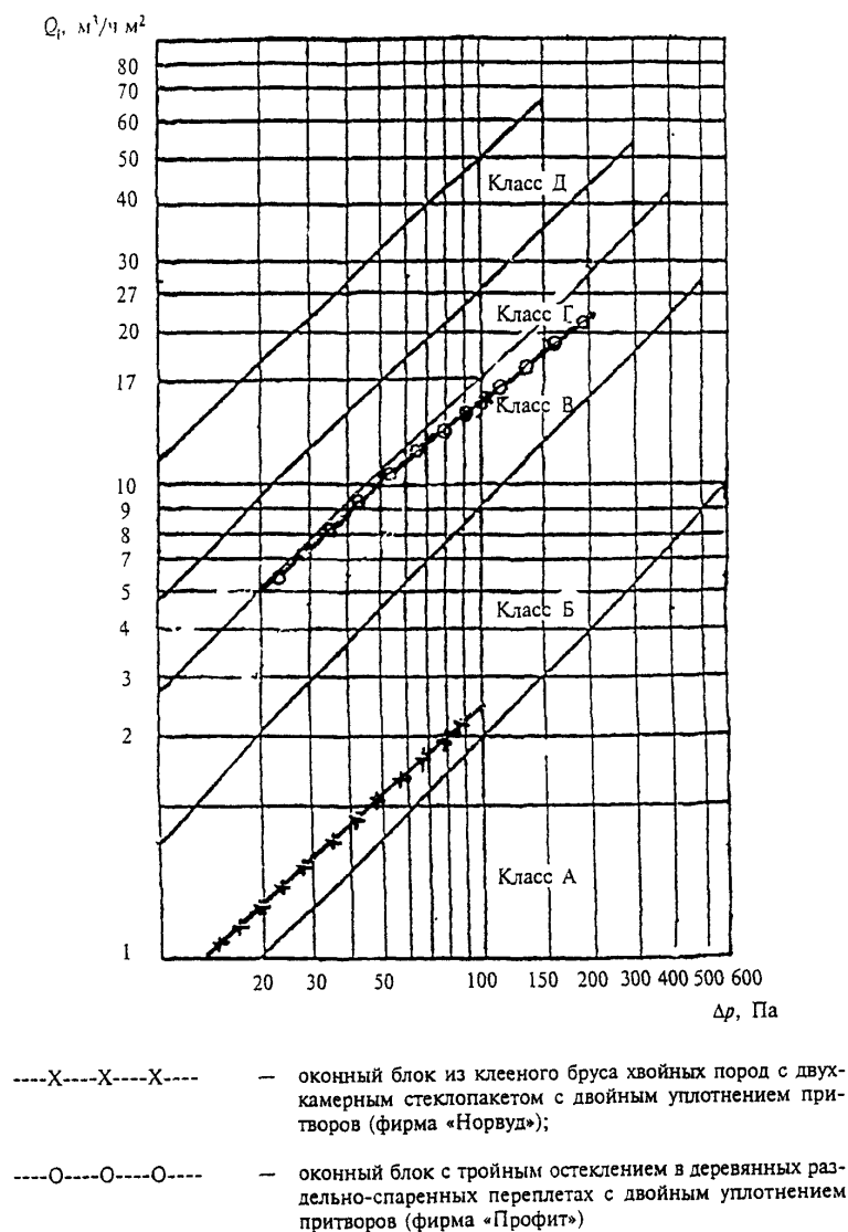
Рисунок Ц.1. Графики зависимостей объемной воздухопроницаемости Q_i от перепада давления \Delta p по результатам сертификационных испытаний оконного блока, сопоставленные с графиками нормативных прямых, определяющих границы классов оконных блоков по воздухопроницаемости по ГОСТ 26602.2.
