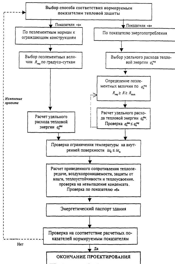
Рисунок 1. Схема проектирования тепловой защиты зданий
