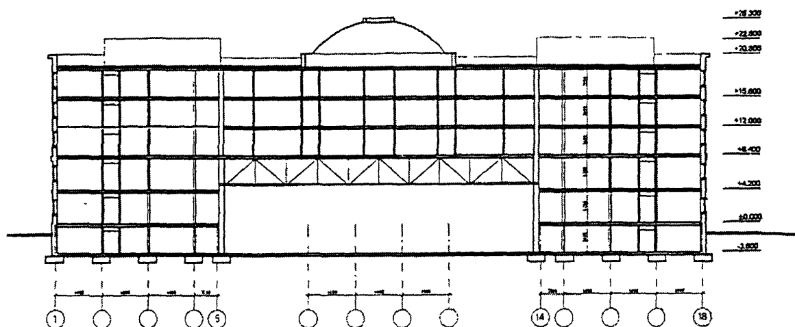
Рисунок Я.3. Продольный разрез
