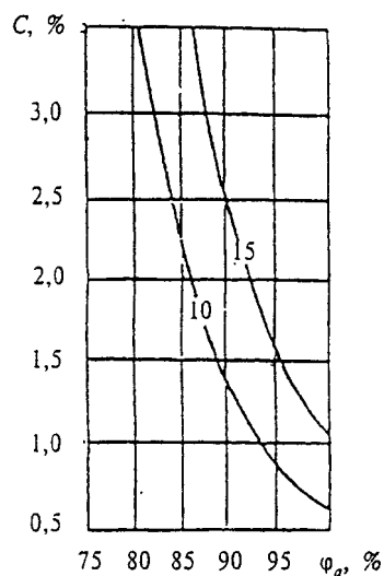
Рисунок Щ.2. Изолинии сорбционного влагосодержания керамзитобетона \rho_0 = 1200 \text{ кг/м}^3 , содержащего хлорид калия, при изменении относительной влажности воздуха \varphi_a , %, и массового солесодержания C , %
