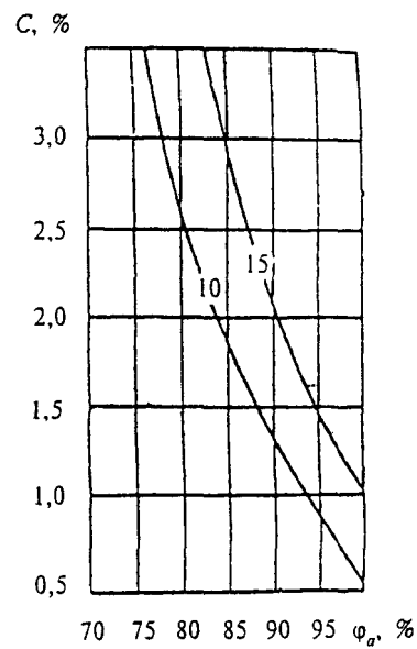
Рисунок Щ.6. Изолинии сорбционного влагосодержания
