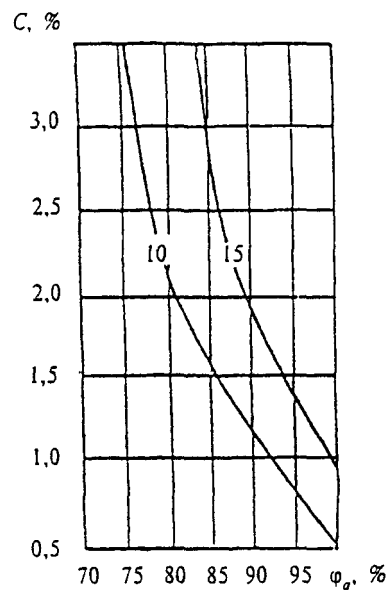
Рисунок Щ.5. Изолинии сорбционного влагосодержания
